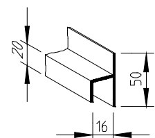
Abschlußprofil
