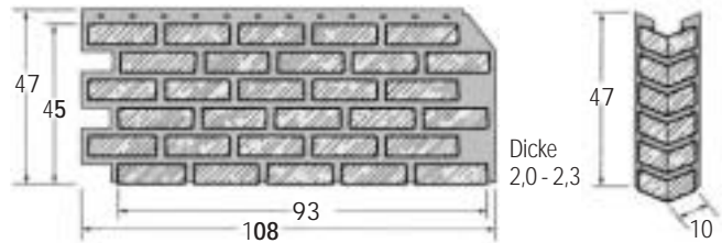
TERRAPRIK-Klinkermuster
